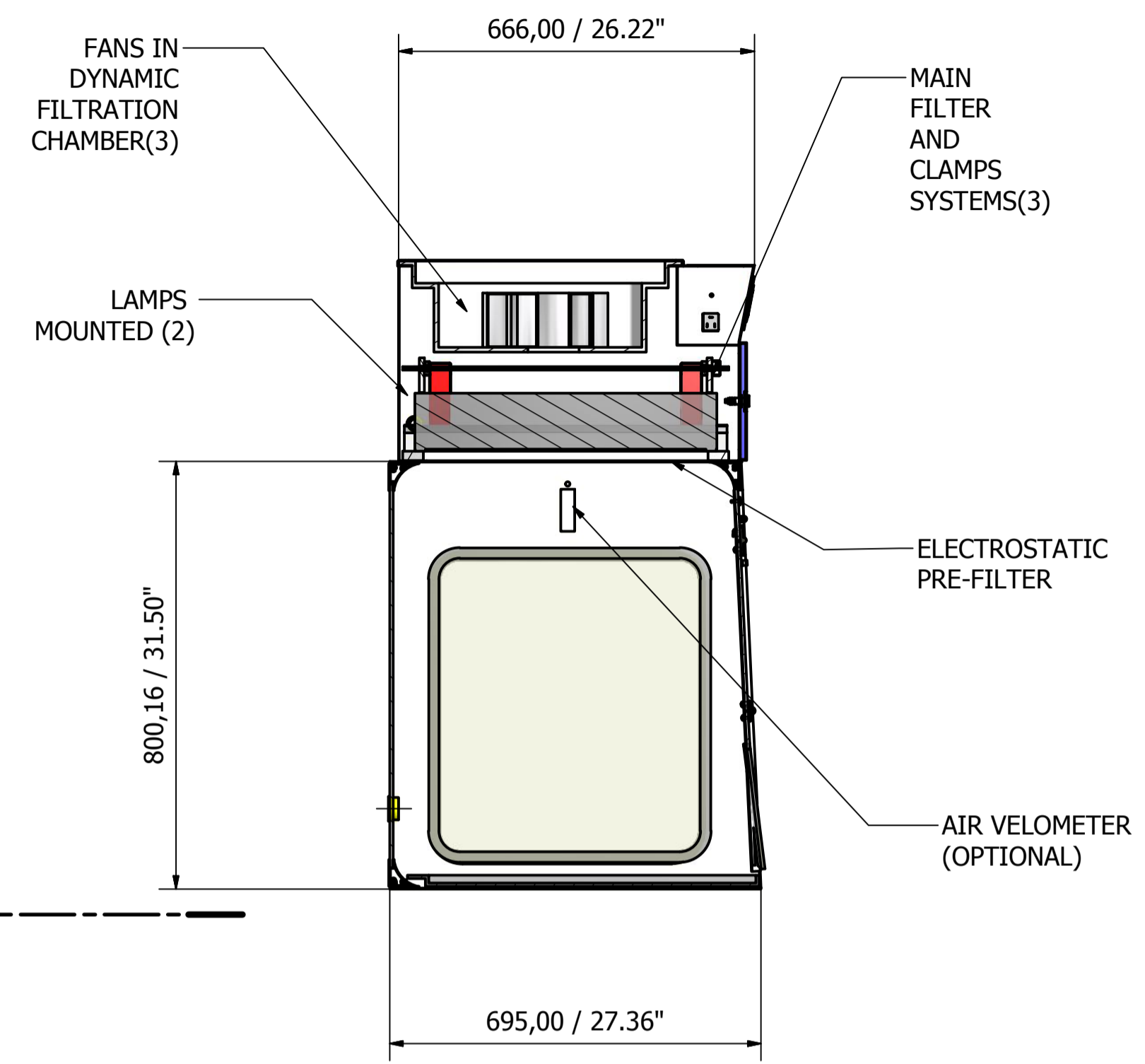
B-B ( 1 : 10 )
