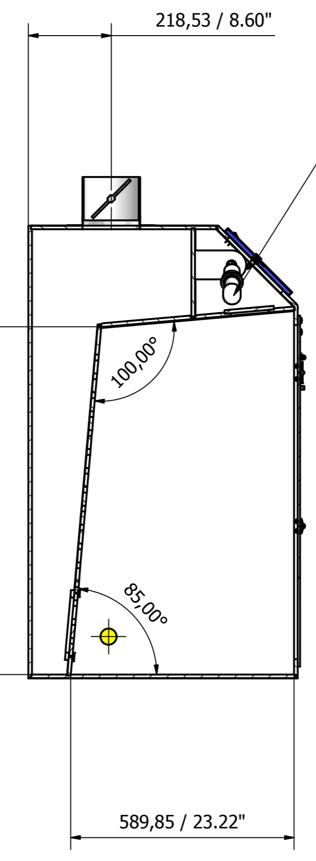
A-A ( 1 : 10 )
