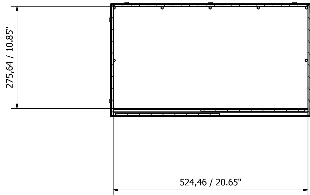
B-B ( 1 : 5 )
