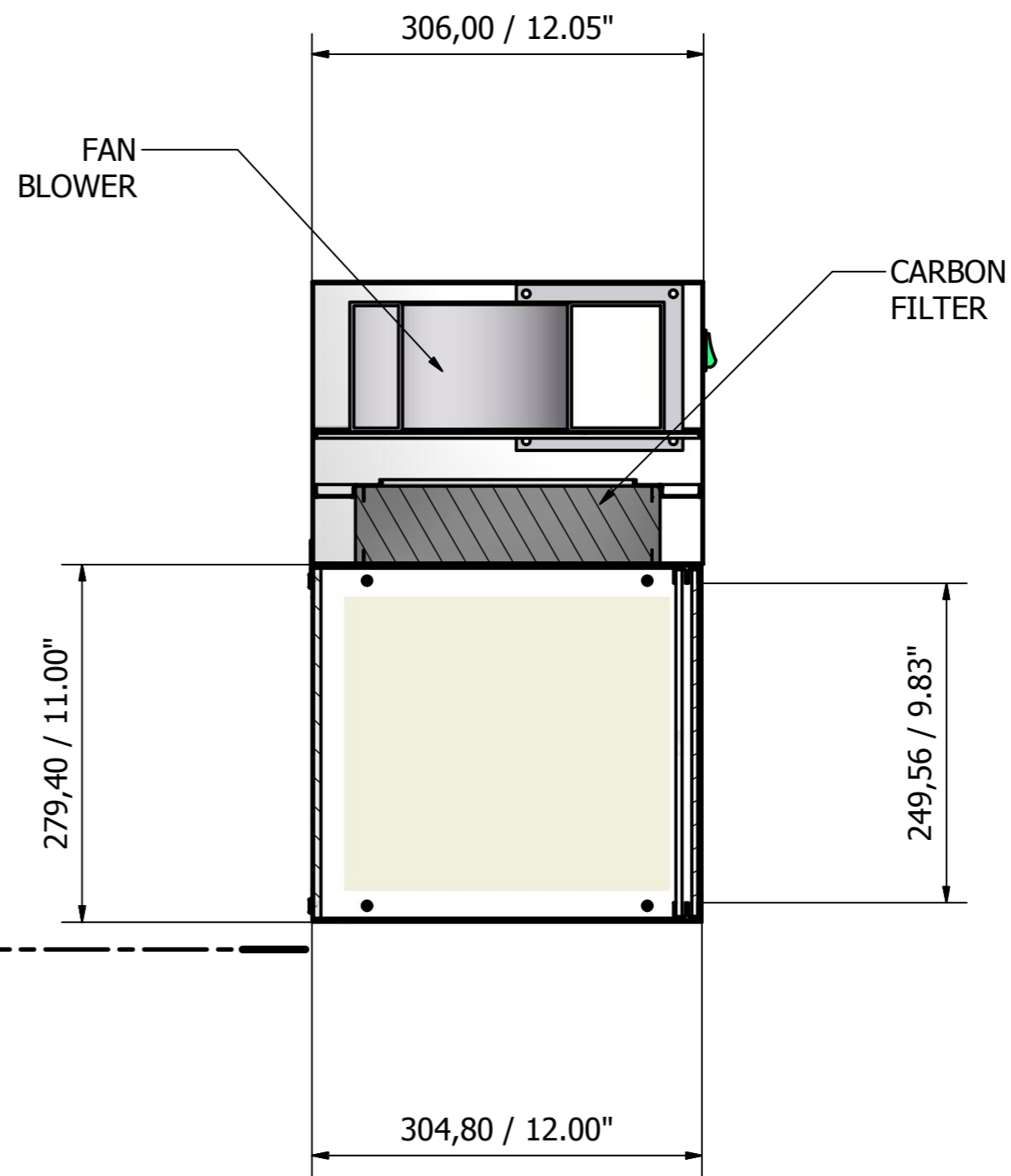
A-A ( 1 : 5 )
