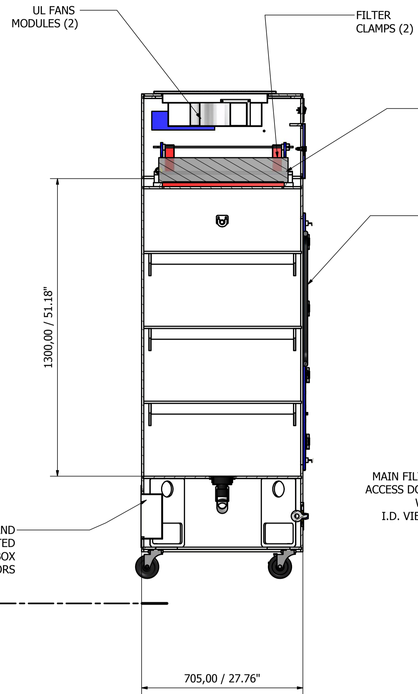
A-A ( 1 : 10 )
